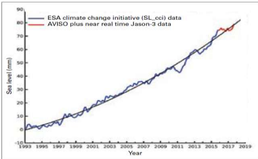
نمودار ۱. میانگین جهانی سطح دریاها طی دوره ۱۹۹۳-۲۰۱۸ (میلیمتر)
