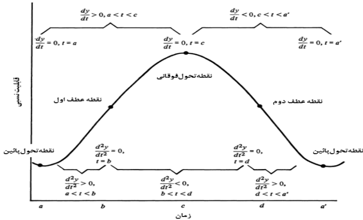
شکل ۱. منحنی عمومی قابلیت نسبی و نقاط بحرانی
